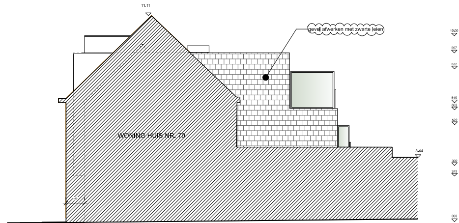
rechterzijgevel
