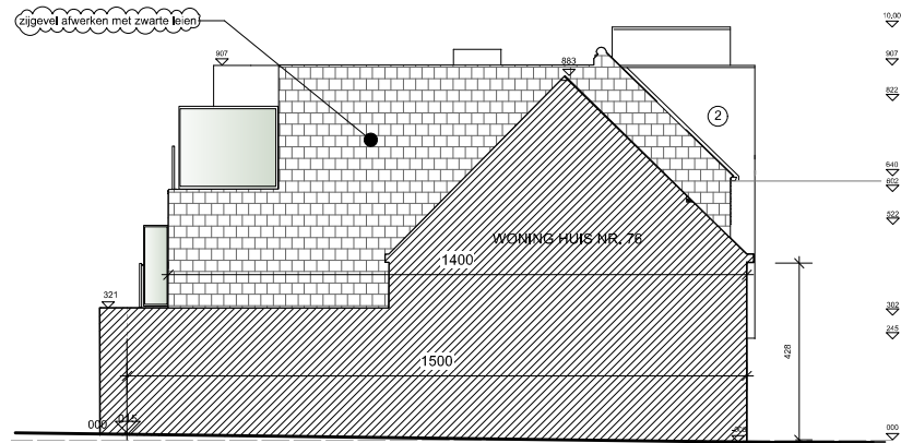
linkerzijgevel
